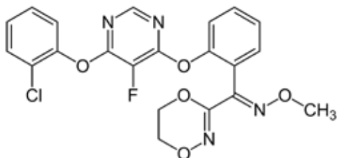
Fluoxastrobin FRAC 11
